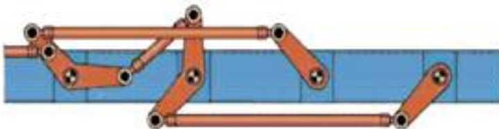
Gestänge für gegenläufige Bewegung
