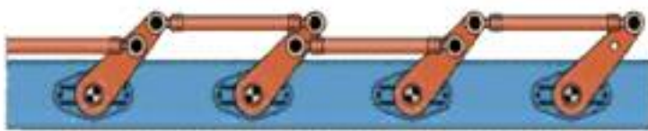
Gestänge für gleichläufige Bewegung
